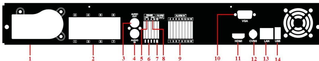
Рис. 2.4. Задняя панель LTV-NVR-1630P
