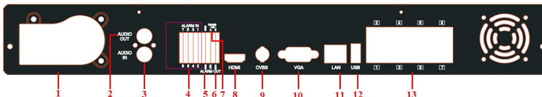
Рис. 2.3. Задняя панель LTV-NVR-0830P
