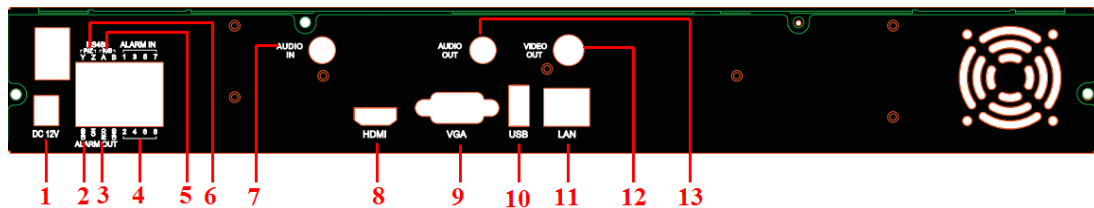
Рис. 2.1. Задняя панель LTV-NVR-0830
