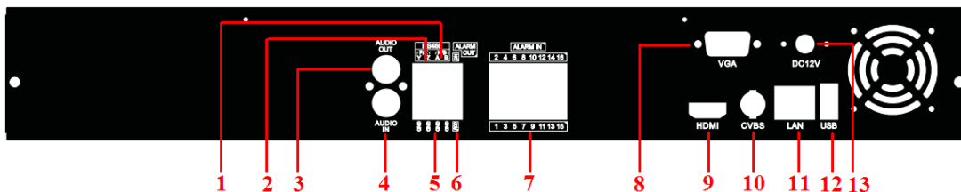
Рис. 2.2. Задняя панель LTV-NVR-1630 / LTV-NVR-1631
